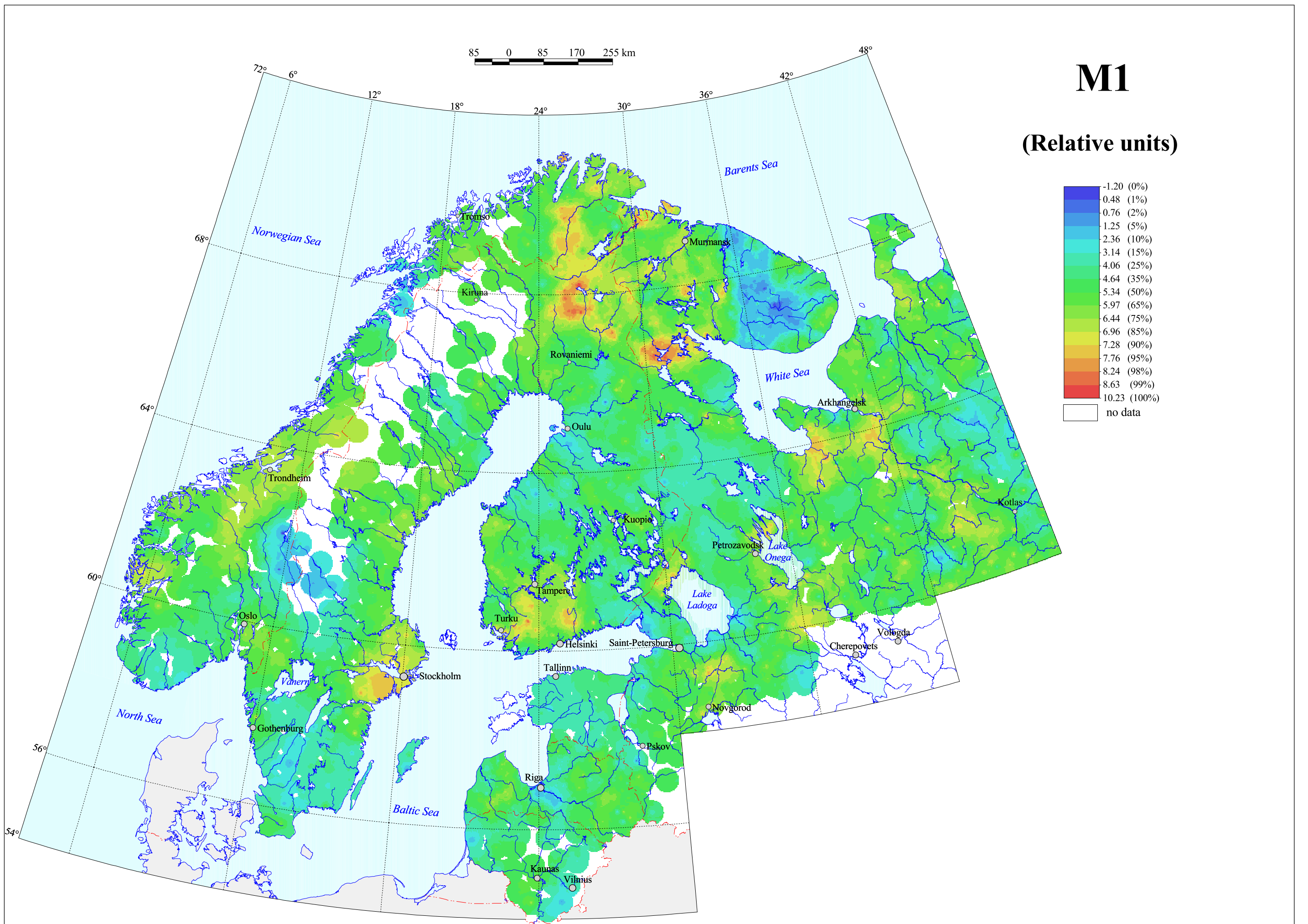
M1 (Co, Cr, Cu, Ni, V) in C-horizon, Grain Size <2 mm, Aqua regia Extraction
